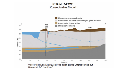
Der rechtsufrige, tiefe Kolk beim Aarwil. (Hydrogeologische Untersuchungen Wehrliau, Universität Neuenburg, Oktober 2024).
